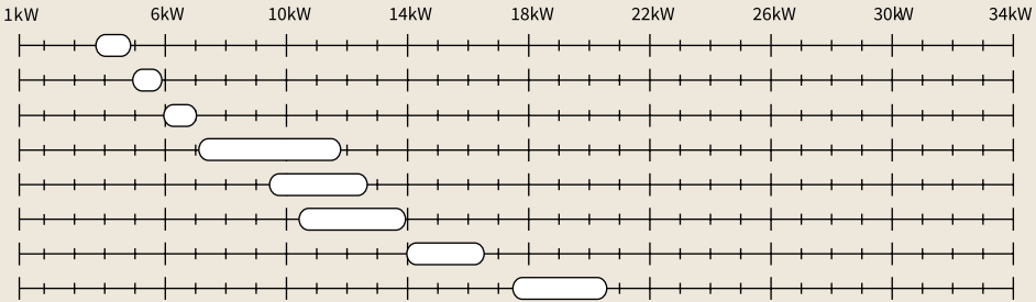
Rango de capacidad de refrigeración en las condiciones: entrada/salida de agua: 12/7 °C; temperatura exterior: 35 °C (DB).
