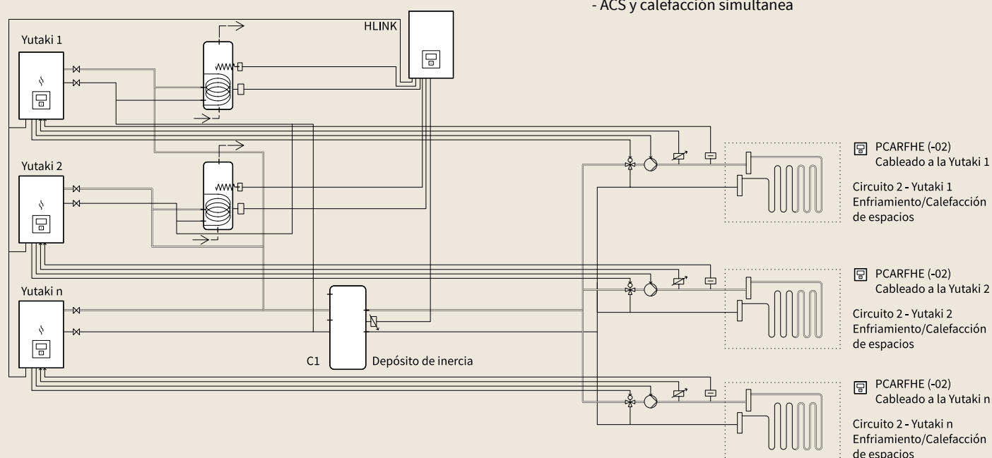
Producción de ACS individual y calefacción en cascada con tres Yutaki
