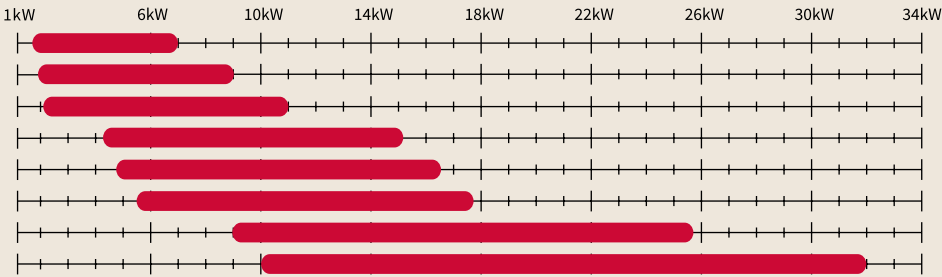
Rango de capacidad de calefacción en las condiciones: entrada/salida de agua: 30/35 °C; temperatura exterior: 7/6 °C (WB/DB).
