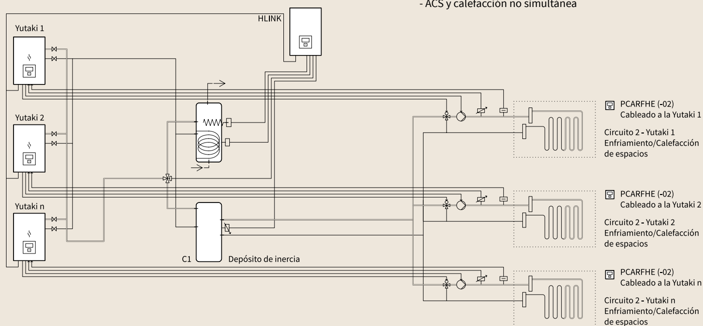
Producción de ACS y calefacción en cascada con tres Yutaki
