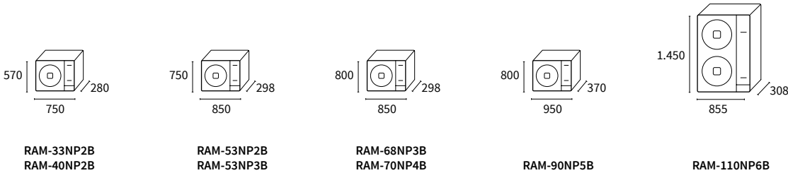
Unidades exteriores
