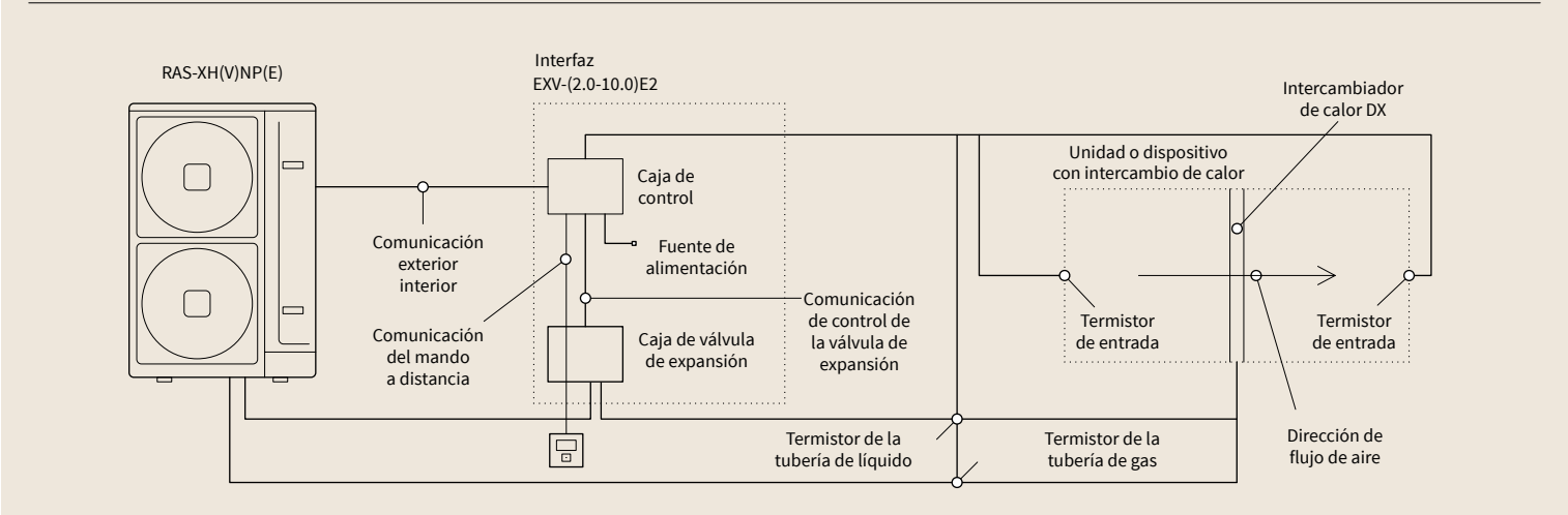
Válvula de expansión y caja de control
