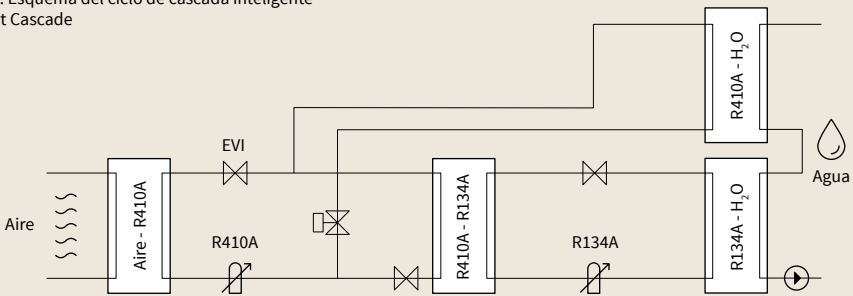
Fig. 1: Esquema del ciclo de cascada inteligente Smart Cascade
