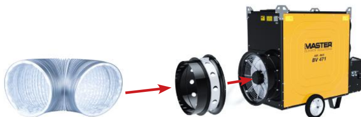
Tubo de succión + Kit de recirculación de aire
